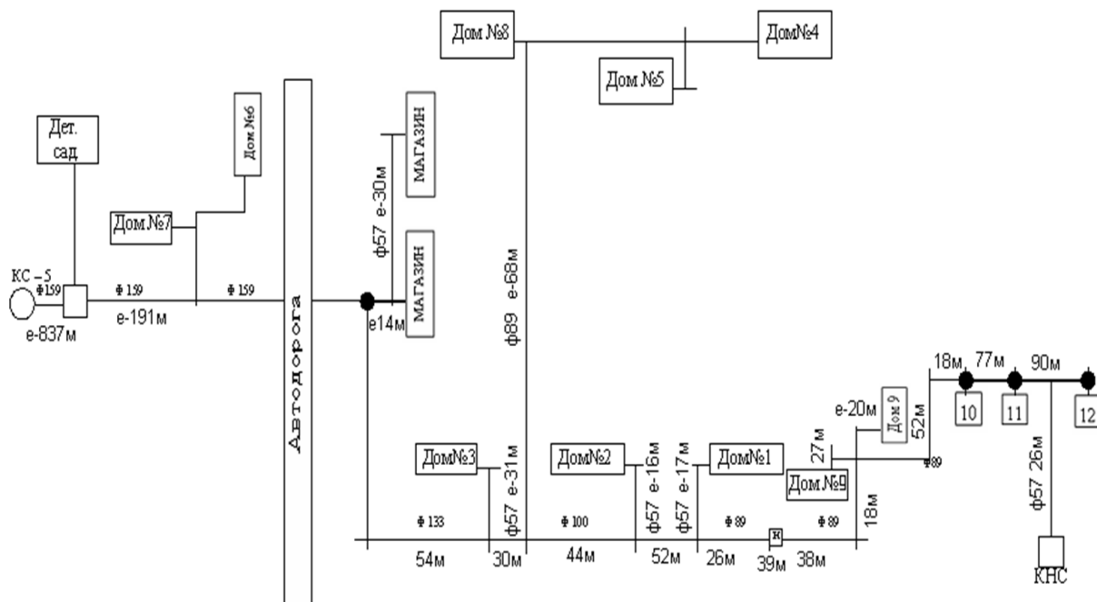
Схема инженерных коммуникаций системы теплоснабжения жилого поселка газодомовиков Акбулым
